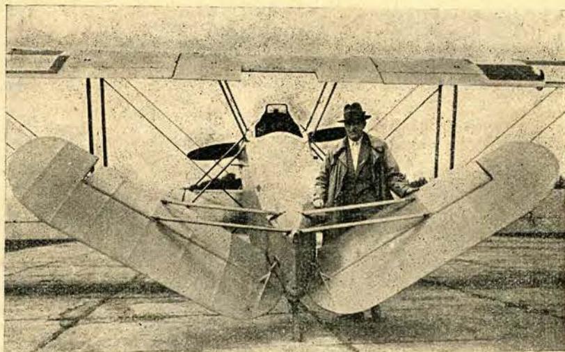
Na lotnisku Mokotowskim demonstrowany był nowy wynalazek sterów samolotowych, skonstruowany w lubelskiej fabryce samolotów. Wynalazek ten polega na tem, że dotychczasowe stery, dwa poziome i jeden pionowy, zastąpione zostały dwoma sterami. Wynalazek ten pozwala na większą zwrotność samolotu oraz wymijanie przeszkód przy lądowaniu.
