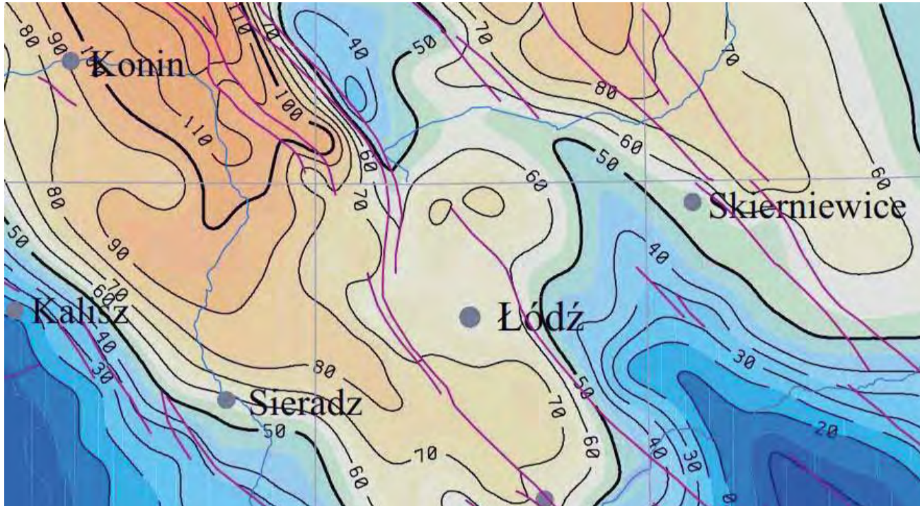
Rozkład temperatur w stropie jury.
