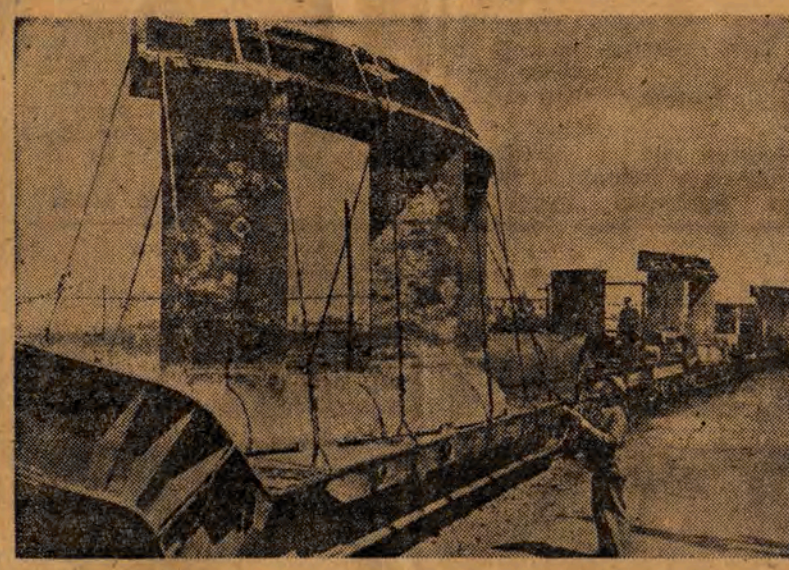
W potężnych elektrowniach — budowanych obecnie w Związku Radzieckim — instalowane zostają gigantyczne turbiny wodne. Zdolność przepustowa tych turbin wynosi kilka tysięcy metrów sześciennych na sek.
