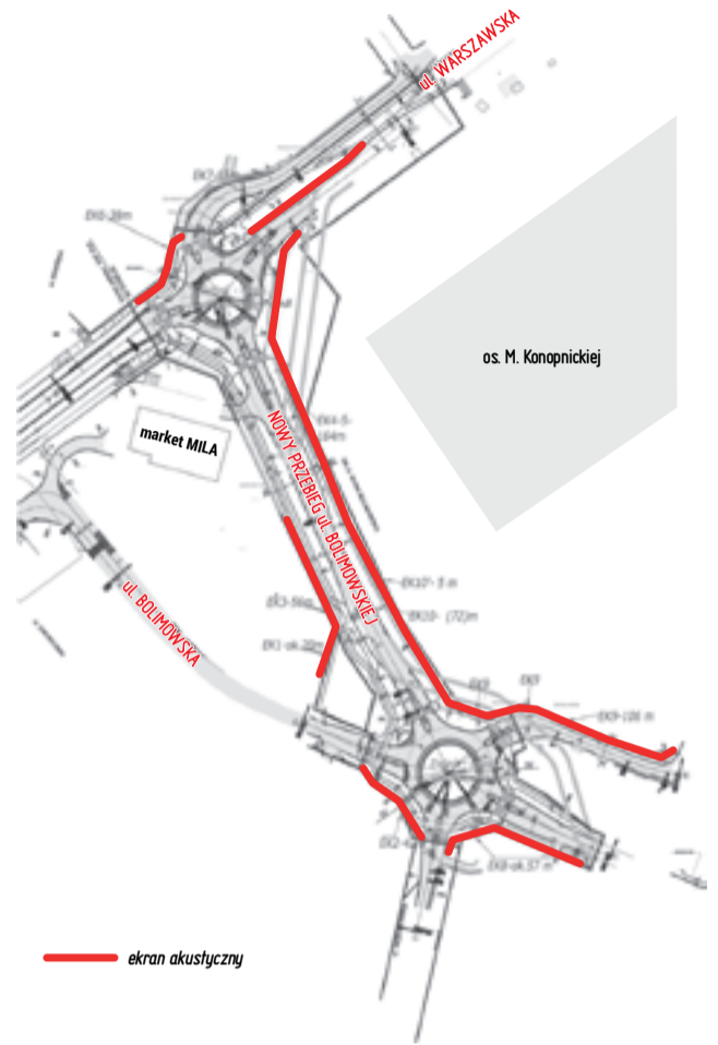
Lokalizacja ekranów akustycznych wzdłuż nowego odcinka ul. Bolimowskiej i w obrębie planowanych dwóch rond.
