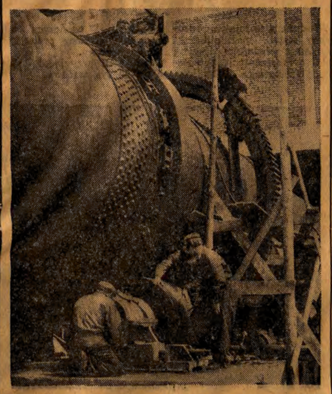
W województwie krakowskim powstaje nowoczesna huta cynku. Urochomienie huty nastąpi jeszcze w bieżącym roku. Założa budowniczych huty podlega szeregowi zobowiązań produkcyjnych celem jej przedterminowego uruchomienia. NA ZDJĘCIU: Brygada ślusarzy-monterów Stanisława Kondusza przeprowadza montaż piece obrotowego do wypalania rudy. CAF - fot. Baranowski
