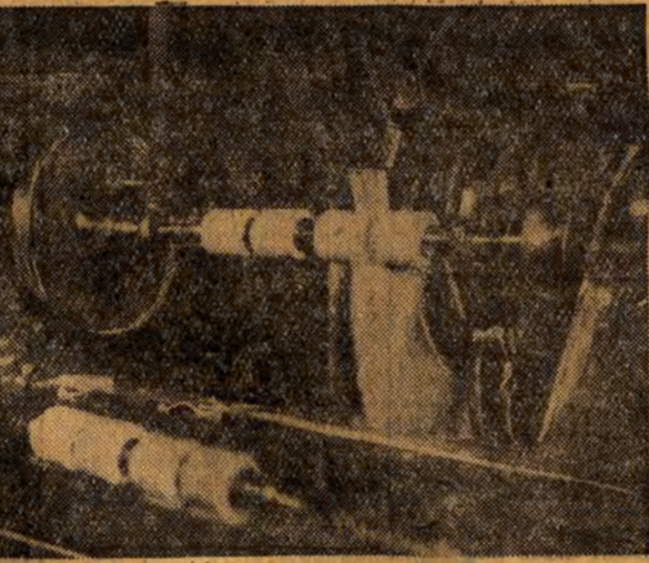
Szlifowanie wałków obciążonych masą plastyczną.
