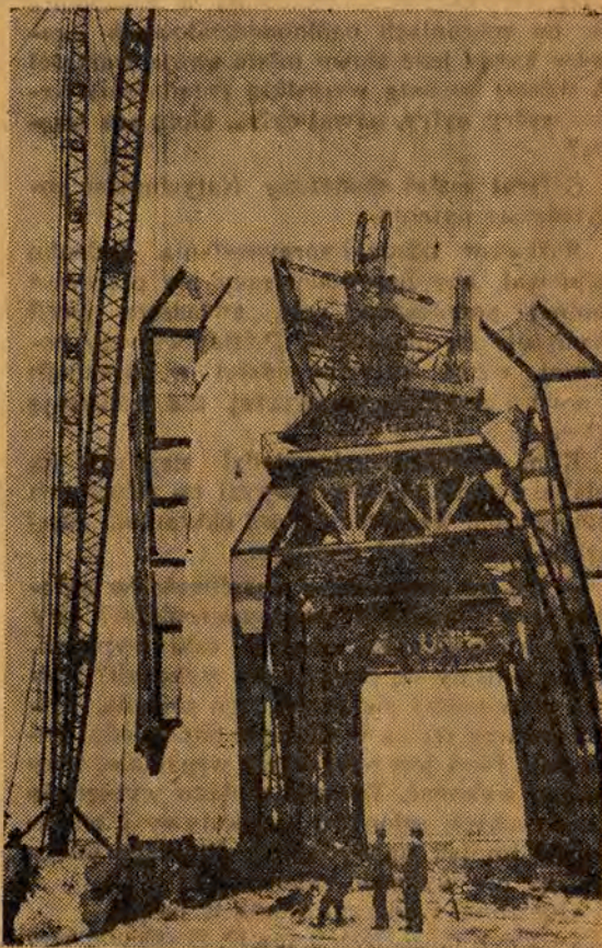
Montaż dźwigu portalowego na jednym z placów budowy Kujbyszewskiej Elektrowni Wodnej. Fot. — CAE
