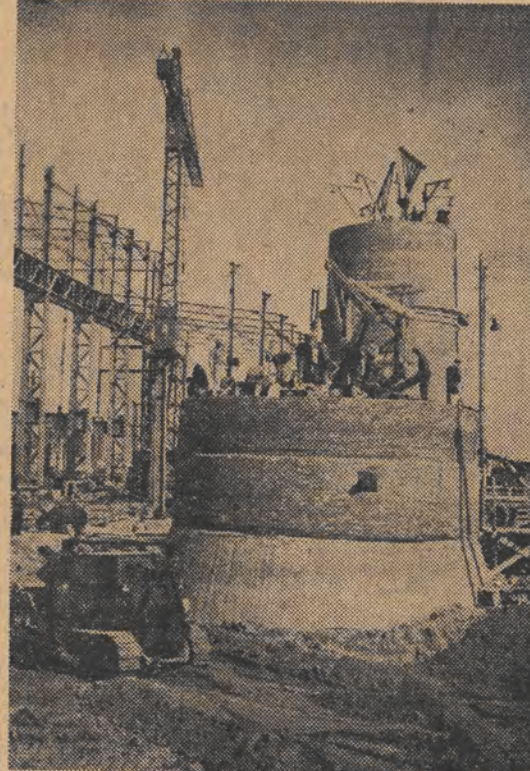
NA ZDJĘCIU: budowa kominów do pieców martenowskich. CAF — fot. Pienkowski
