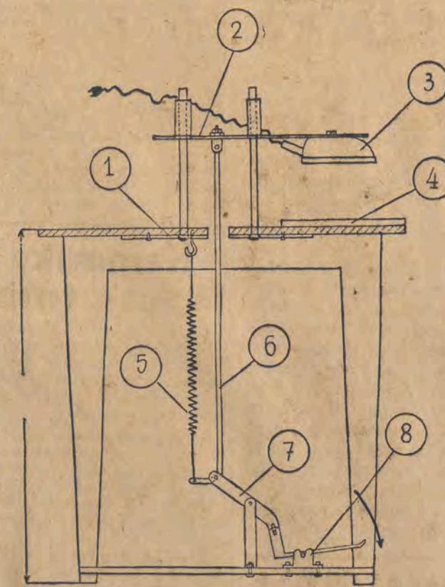
Schemat maszyny do stemplowania półoczek — pomysłu ob. Kotlickiego
