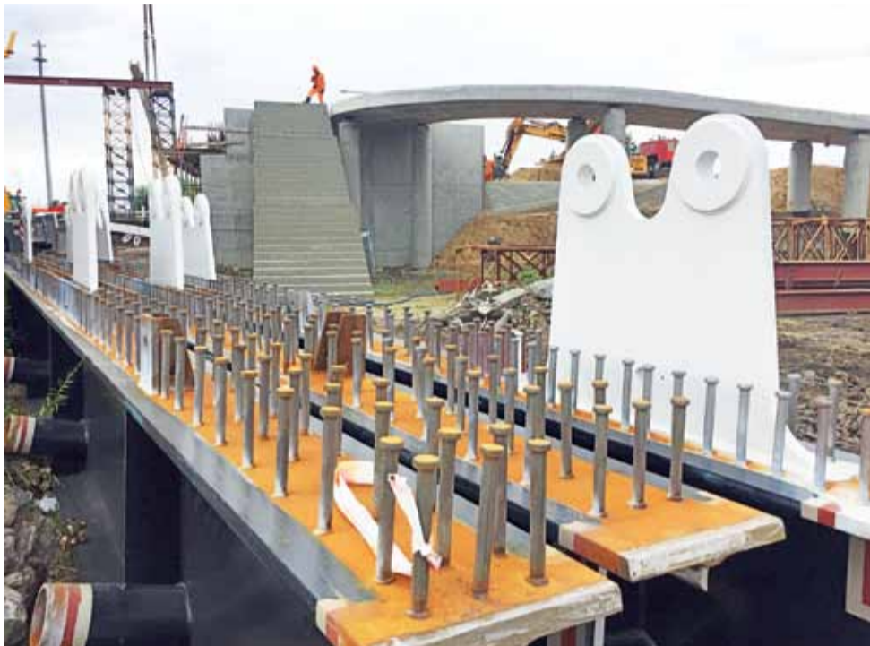
Belki przyszłej jezdni. Widać zaczepy lin nośnych.
