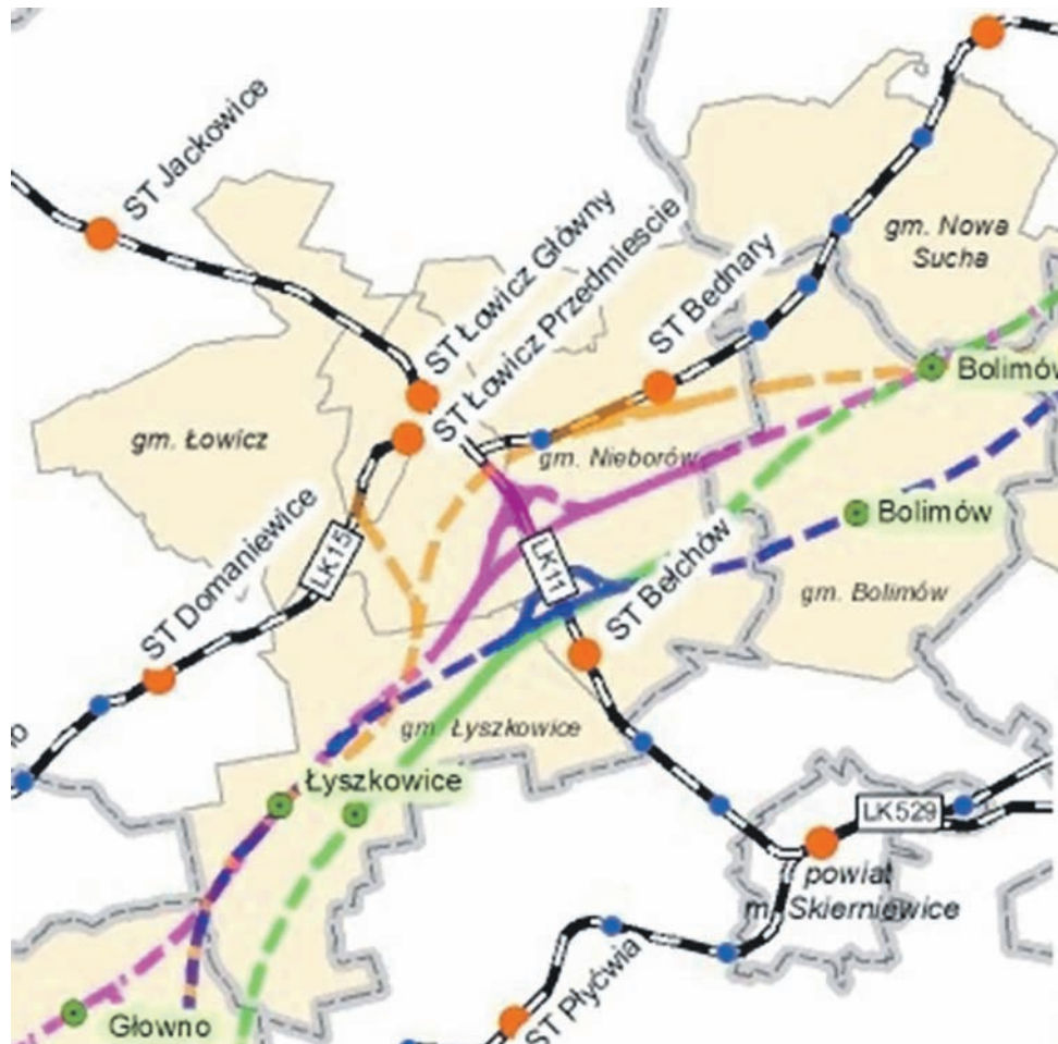
Przebieg projektowanej linii kolejowej nr 85 oraz istniejącej infrastruktury kolejowej.
