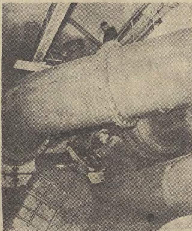
Rurociąg Pilica — Łódź to nie tylko same rury ułożone na 48-kilometrowej trasie. To również wiele budownictwa i najprzeróżniejszych gigantycznych urządzeń. Oto na przykład fragment halli pomp wysokiego ciśnienia.
