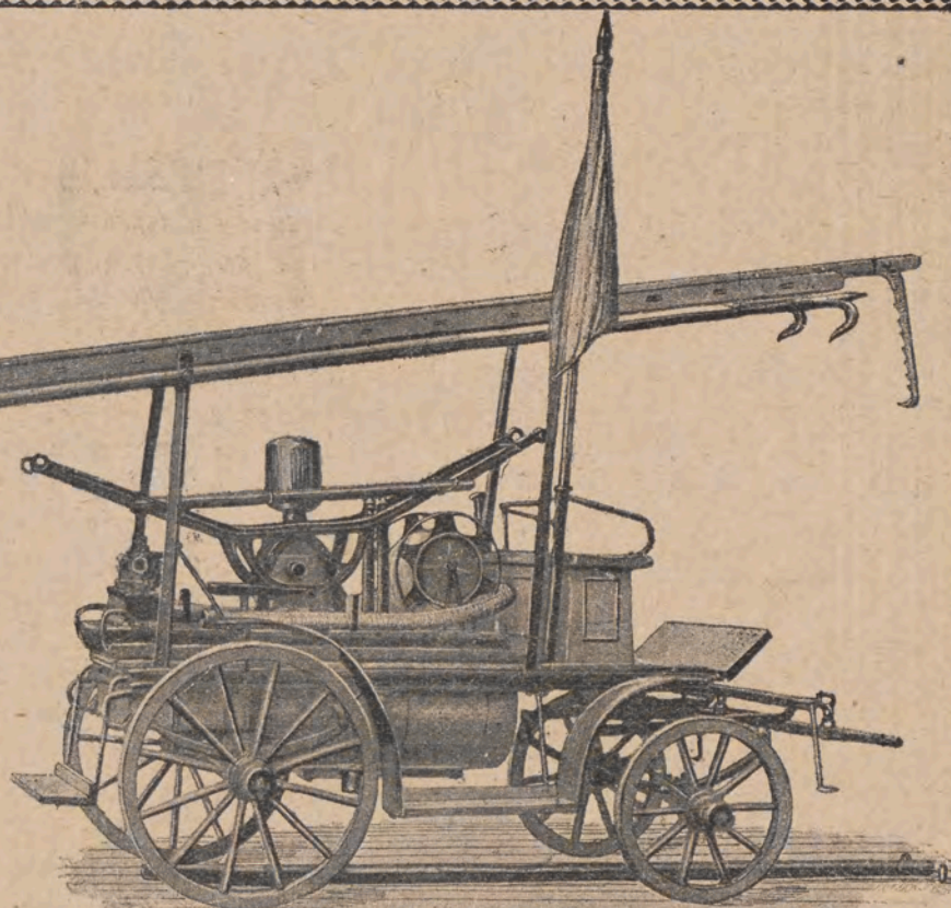
Wóz pogotowia wodnego ze zbiornikiem, pojemności 300 litr. i sikawką zdejmowaną „Tryumf”.
