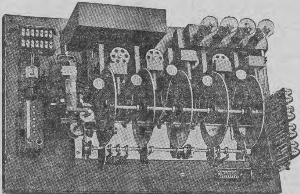
Mechanizm zegarowy, zainstalowany i uruchomiony w gmachu P. A. S. T., który w odstępach 10 sekundowych nadaje telefonicznie dokładny czas.
