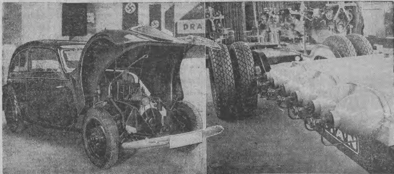
Na lewo: Wóz, w którym jednym ruchem podnosi się maskę, obnażając cały motor. Na prawo: Podwozie auta, poruszanego sprężonym powietrzem.
