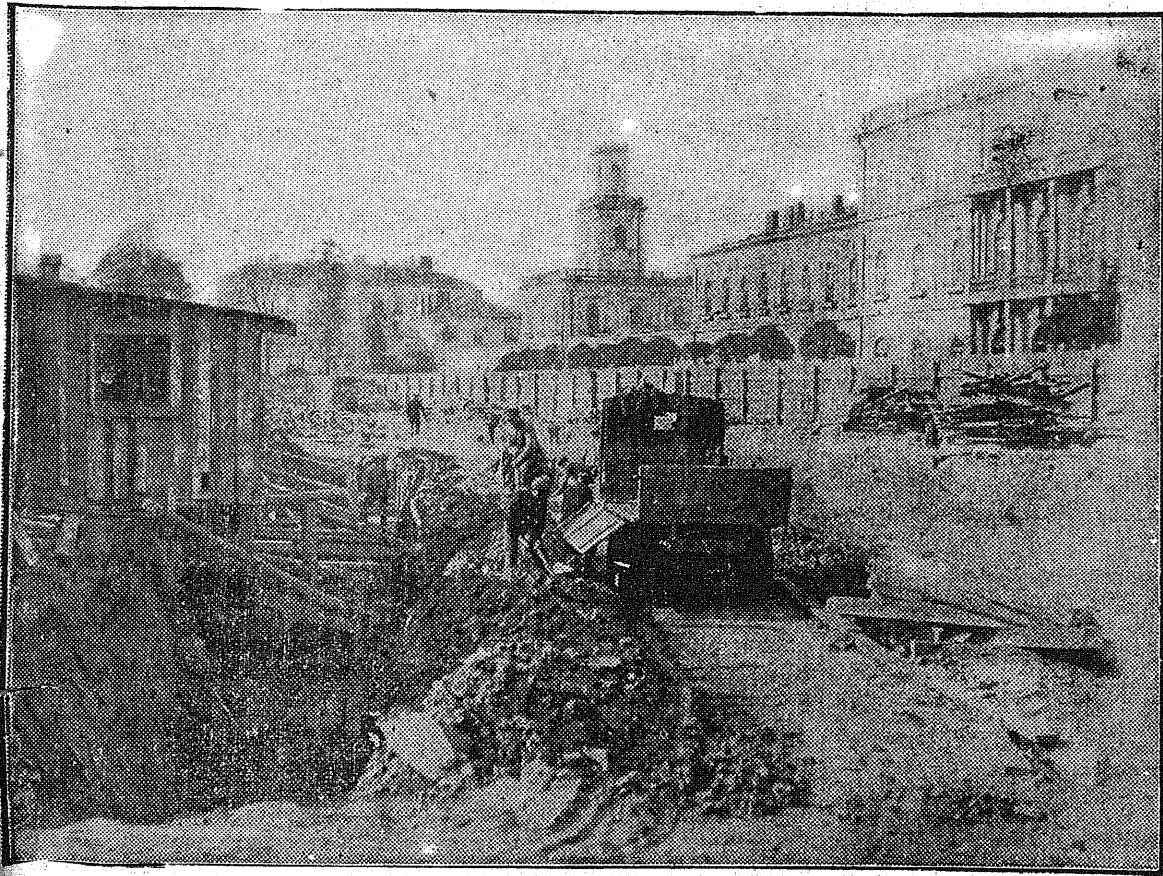
Obok dworca głównego, na skrzyżowaniu dwóch ważnych arterji, ul. Marszałkowskiej i Al. Jerozolimskiej, trwa praca nad budową tunelu kolejowego. Jest to ostatni etap prac, prowadzonych w centrum największego ruchu kołowego i pieszego.
