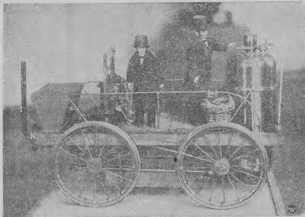
Reprodukujemy zdjęcie ze zbiorów Szwedzkiego Muzeum Technicznego w Sztokholmie przedstawiające autentyczny wynalazek Jana Ericsona, a mianowicie pierwszą jego lokomotywę, typu „Novelty”.
