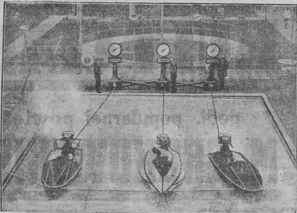
Wycigowe łodzie motorowe przymocowane są stalowymi linami do aparatów pomiarowych, które określają szybkość, regularność jazdy i wytrzymałość puszczonych w ruch silników.
