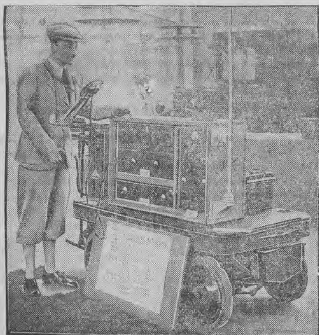
RUCHOMA STACJA NADAWCZA znajduje zastosowanie przede wszystkim przy reportażach.
