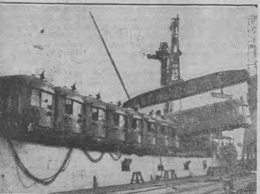
Transport elektrowozów, załadowanych na okręt w Bristolu.
