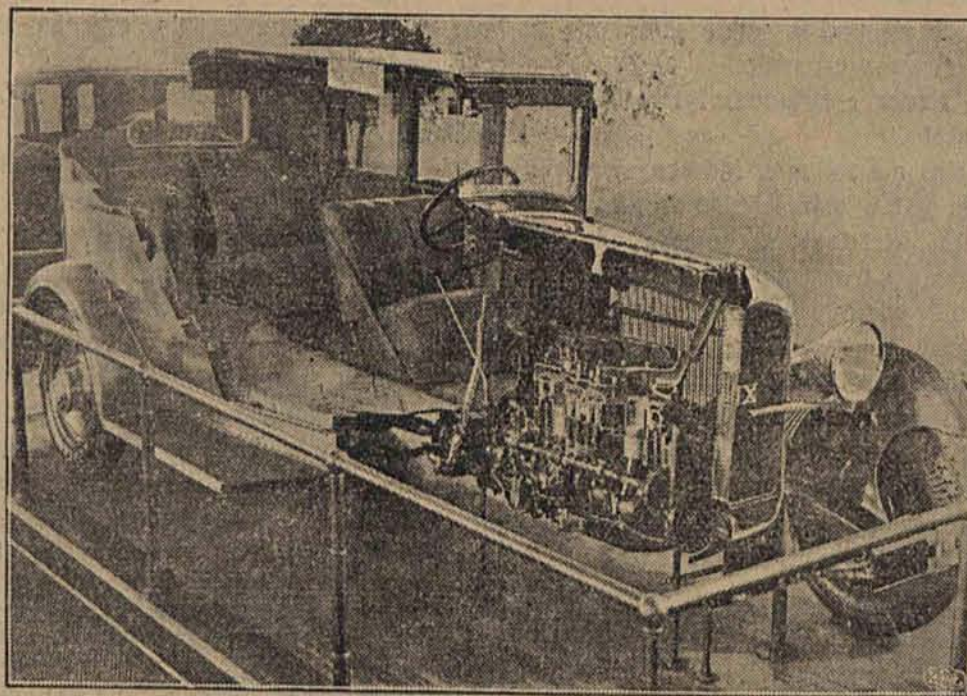
Przekrój samochodu Citroën zwraca uwagę fachowych automobilistów, zwiedzających Wystawę Samochodową Citroën w Warszawie.
