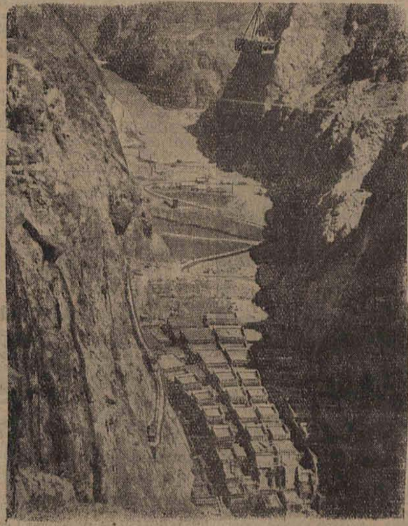
Tama Hoovera w południowej Kalifornii zasługuje bezsprzecznie na nazwę największego cudu świata. Trwające już oddawna prace przeciągną się prawdopodobnie 10 lat i koszt ich wyniesie 387 milionów dolarów. Ilustracja powyższa przedstawia stan robót nad budową tej tamy.
