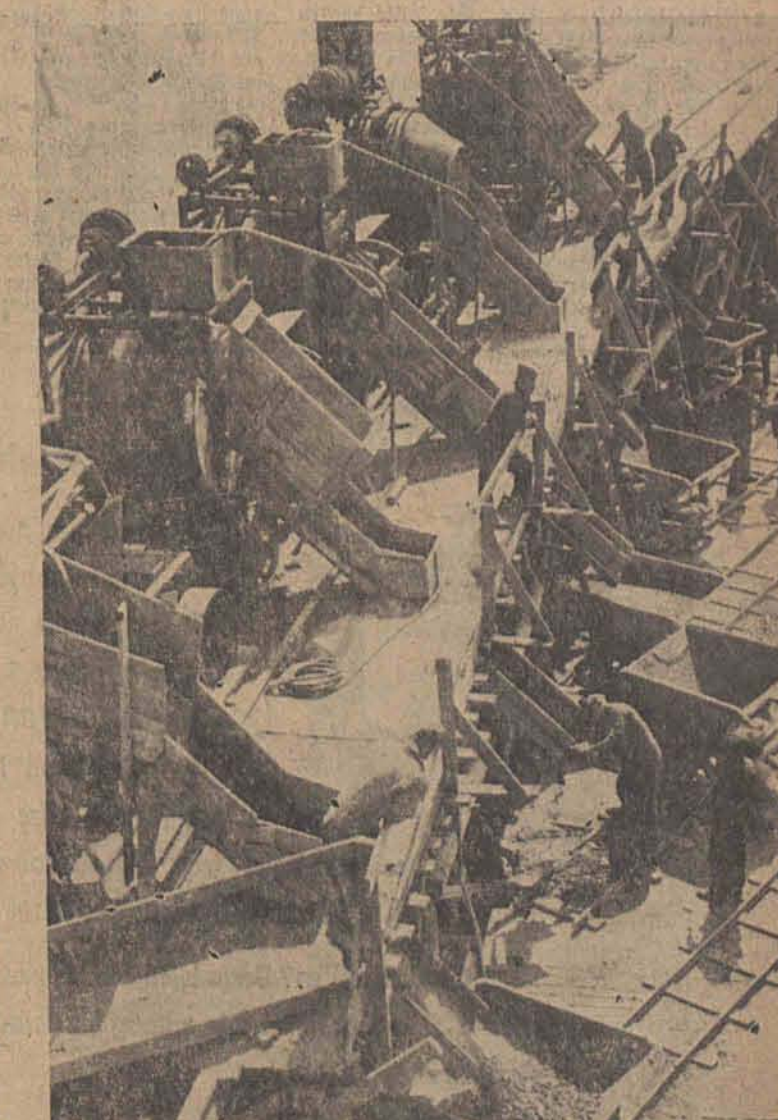
Menschen und Maschinen der Organisation Todt an der Front schaffen gegen England Links: Eisenflechter bereiten das Gerüst. Rechts: In langen Reihen stehen die Beton-Mischmaschinen. Auf der einen Seite rollt das Material heran, auf der anderen verläßt die Betonmasse die Maschinen. Unermüdet arbeiten Menschen und Motoren. Aufn.: O.T. Desau, Brecke-Hoffmann.)
