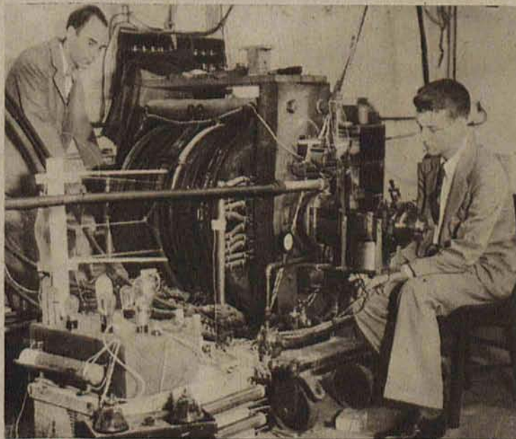
W instytucie technicznym uniwersytetu Pasadena (Kalifornja) udało się poraz pierwszy uwidocznic dla oka elektrony i jony. Są to najmniejsze cząstki materji z których się składa wszystko począwszy od człowieka a skończywszy na gwiazdach.
