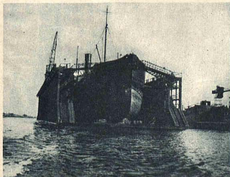
Dok pływający stoczni gdańskiej.
