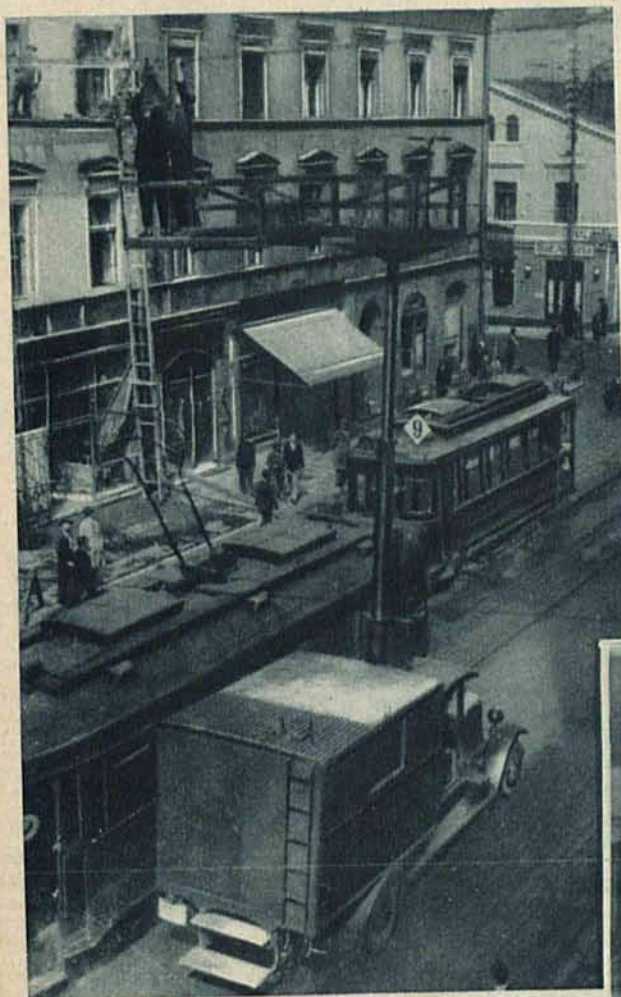
Naprawa przewodów elektrycznych za pomocą nowoczesnych wozów reperacyjnych.
