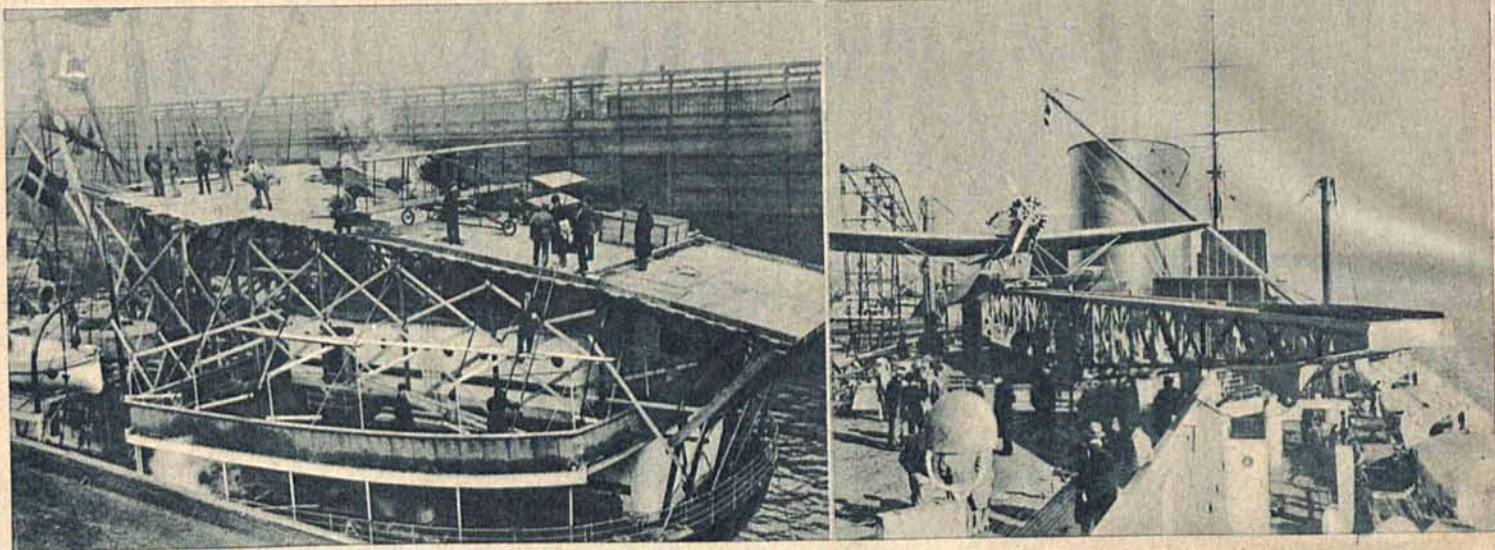
Powyższe zdjęcia wykazują postęp techniki jaki zastosowano przy starcie samolotów pocztowych z pokładu jadącego okrętu. Na lewo start w r. 1910 wymagał olbrzymiego rusztowania i przygotowań w przeciwieństwie do okrętu Bremen, który wysłał samolot przy pomocy urządzenia katapultowego.
