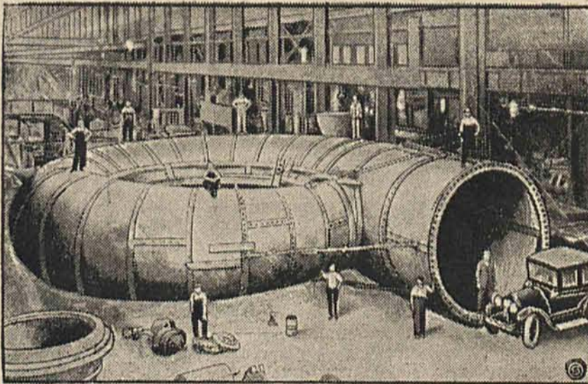
NAJWIĘKSZA TURBINA ŚWIATA Wielkie zakłady budowy maszyn „Hudson Street” w Brocklynie zbudowały ostatnio olbrzymią turbinę o sile 80.000 kilowatów. Kondensator tej turbiny waży około 500 tonn. Posiada on 12.920 rur. Dwie elektryczne pompy poruszające się z siłą 500 koni parowych tłoczą wodę do kondensatora.
