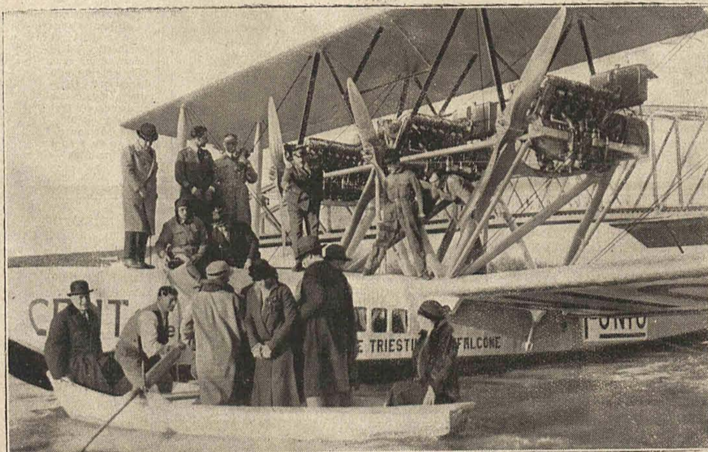
Trójmotorowy aeroplan, utrzymujący stałą komunikację pasażerską między Genuą i Tryjestem
