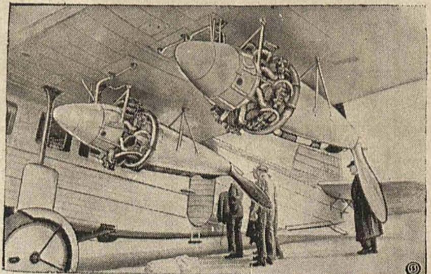
Zdjęcie nasze przedstawia 2 motory nowego statku powietrznego „Kondor” przeznaczony dla lotów na dużych przestrzeniach wystawione w Berlinie podczas ostatniej wystawy aeroplanowej. Mieści on 11 pasażerów i 2 pilotów.
