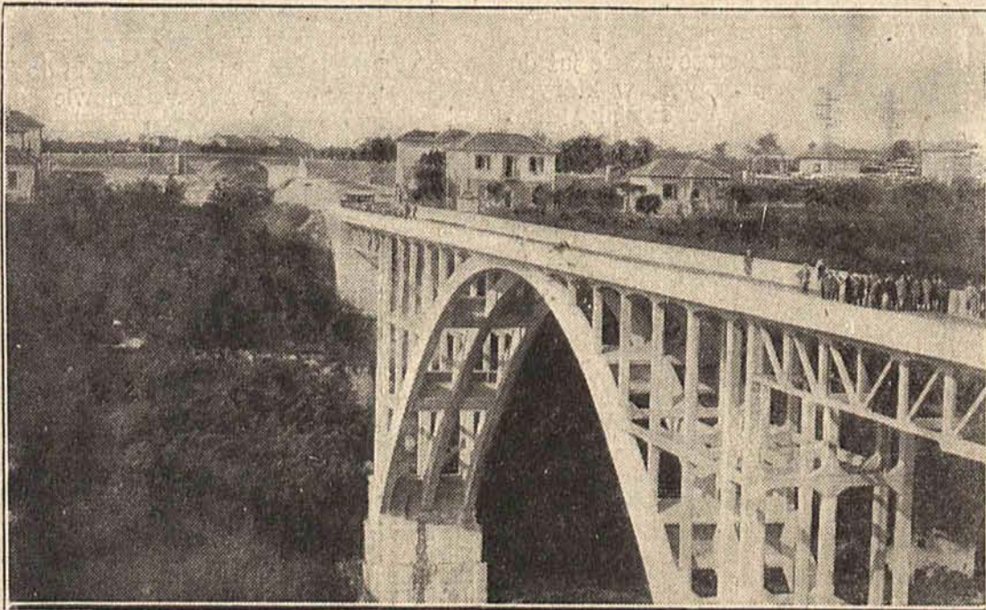
We Włoszech poświęcono przed kilku dniami na drodze pomiędzy Trezzo a Capriate piękny most żelazobetonowy na Adydze. Most ma długości 70 m., a rozpiętość łuku spodniego 80 m.
