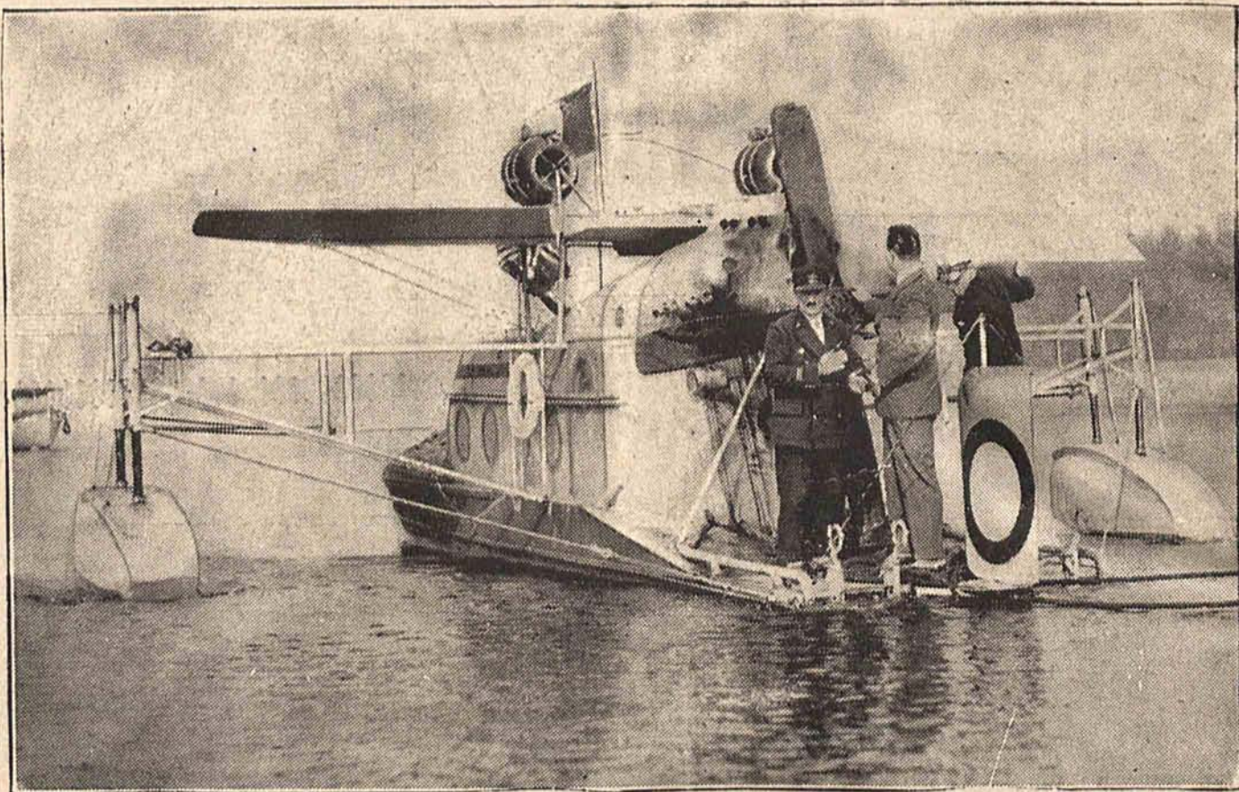
Inż. Bugatti, paryżanin, skonstruował osobliwą maszynę „hydro-skivolator”, czyli połączenie łódki podwodnej, ślizgowca i hydroplanu, która ma służyć mu do przebycia Atlantyku z Havru do New-Yorku z szybkością 100 klm. na godz.
