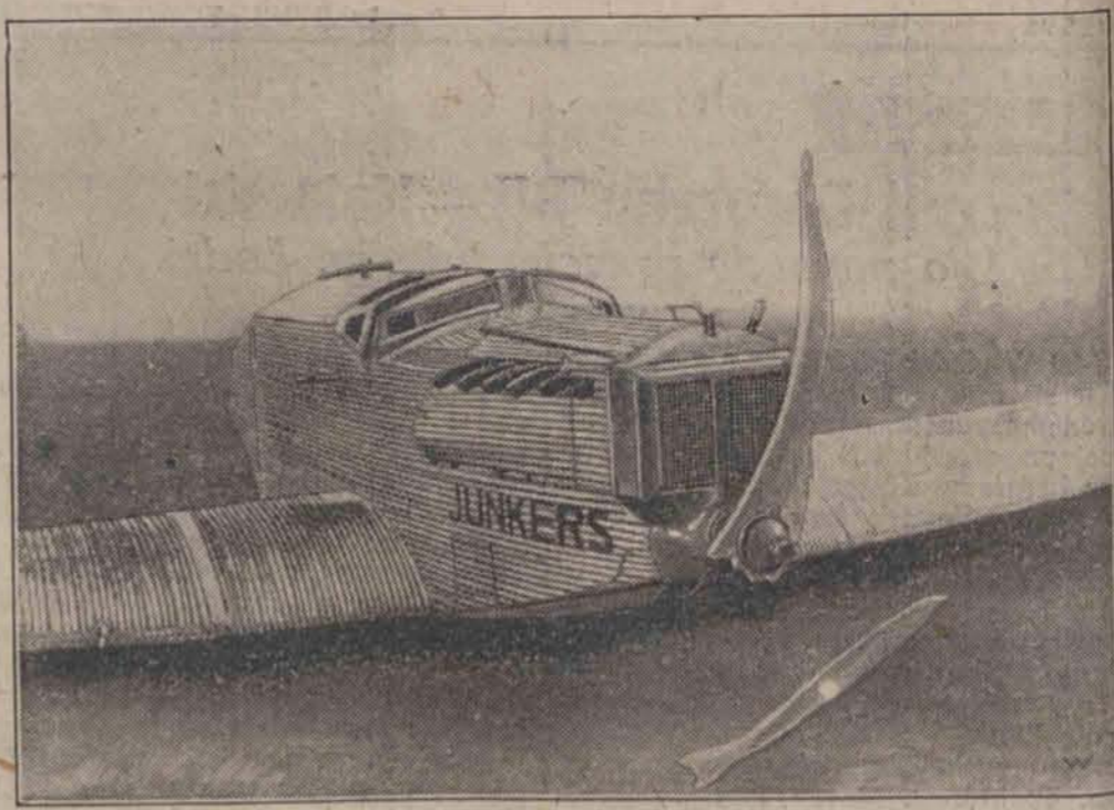
Transatlantyczny samolot „Europa”, który podczas przymusowego lądowania w Bremie uległ częściowemu zniszczeniu. Na zdjęciu, dokonanem tuż po wylądowaniu widzimy złamane śmigło.
