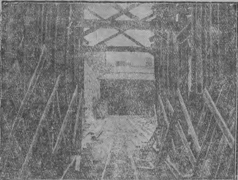
Rusztowanie ustawione pod konstrukcją żelazo-betonową dla pokrycia sklepieniem wylotu tunelu.
