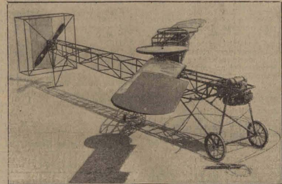
Na lotnisku berlińskim przeprowadzają obecnie próby nowego aparatu, który umożliwia wznoszenie się pionowe z najmniejszej powierzchni bez rozpedu.
