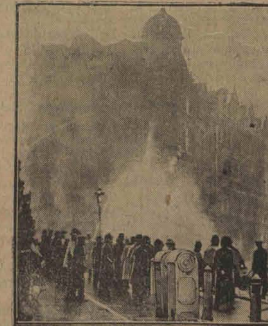
Zwalczanie pożaru.
