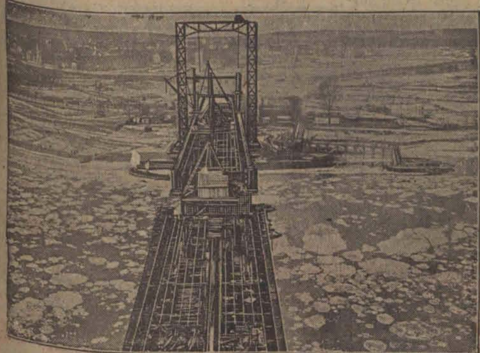
Nad Renem w Kolonii zaczęto przed rokiem budowę nowego gigantycznego mostu, którego jezdnia znajdować się będzie 69 metrów nad poziomem wody. Obecnie Ren ruszył i olbrzymie kry tak uszkodziły filary, że niedokończony most musi ulec rozbiórce. (w)
