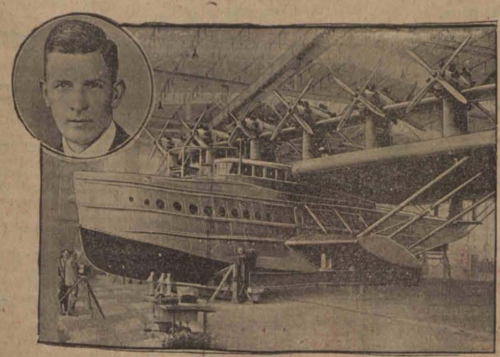
Widok kilku podwójnych motorów, które w sumie reprezentują siłę 6200 KM. Długość 250 kilometrów na godzinę. W sferach fachowców wybudowanie tego aparatu uważane jest za epokowe zdziwienie w dziejach lotnictwa.
