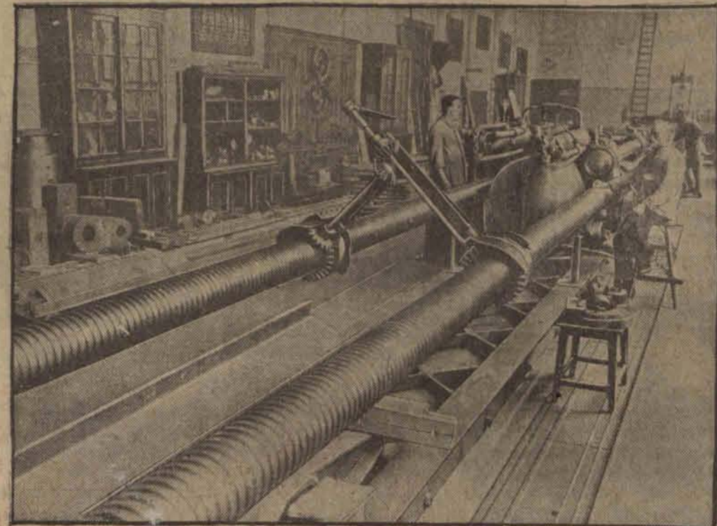
Specjalna maszyna w laboratorium chemicznym do łamania i rozdzielania wałów stalowych wagi do 500 tonn, w celu wyrobowania wytrzymałości materiału. (h)
