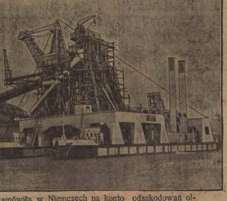
Francja zamówiła w Niemczech na konto odszkodowań olbrzymią dragę parową, która jest największym bogiem świata. Spoczywa ona na dwóch pontonach, wysokość jej wynosi 34 metry. Wiadra mogą w jednej godzinie wybrać z dna morskiego 450 metrów kubicznych ziemi. Draga została przewieziona do portu w Rouen. (w)
