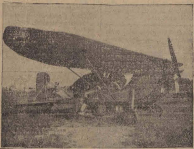
W Touquet we Francji, odbyło się uroczyste święto lotnicze. W czasie tego święta został zaprezentowany nowy typ samolotu jednoosobowego, konstrukcji inż. Desse-nis. Samolot ten o sile motoru 40HP, posiada szybkość 120 km. na godz., przy przeciętnej 90 km. Rozpiętość skrzydeł samolotu wynosi 13 mtr. Samolot zużywa w czasie dwugodzinnego lotu 10 litrów paliwa. Koszt samolotu wynosi około 4 tysięcy złotych.
