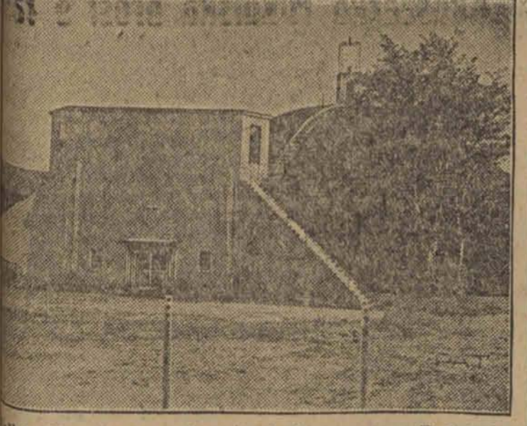
Wielki zbiornik na wodę w wybudowany przez Państwowe Zakłady Wodociągowe.
