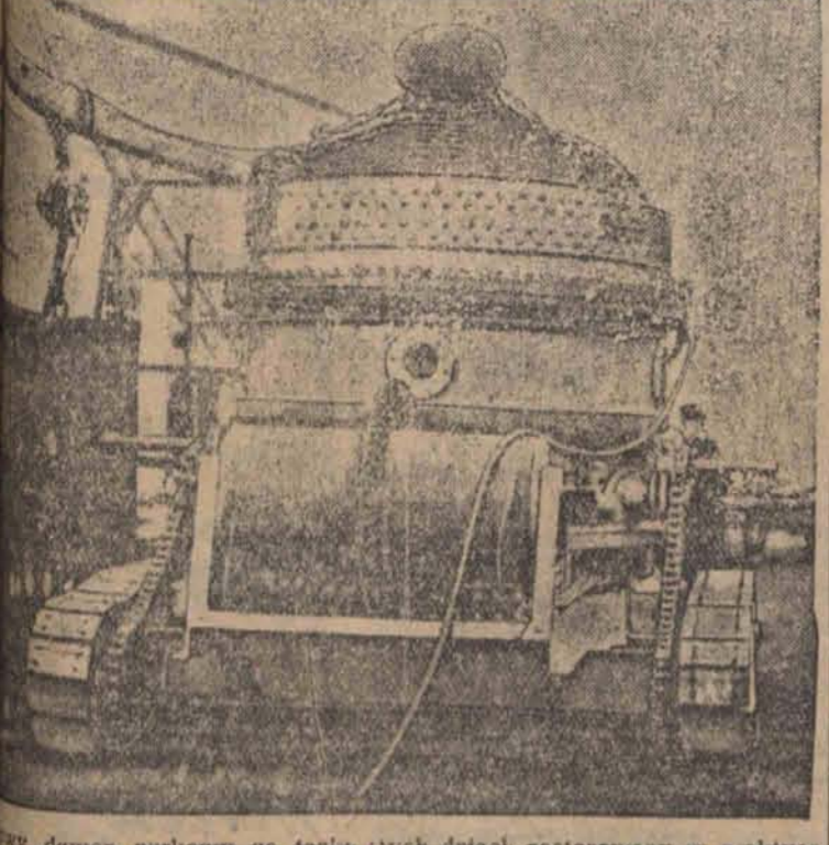
Widok z przodu pierwszego tanku podwodnego, który został po raz pierwszy w 1900 r. w Nowym Jorku.
