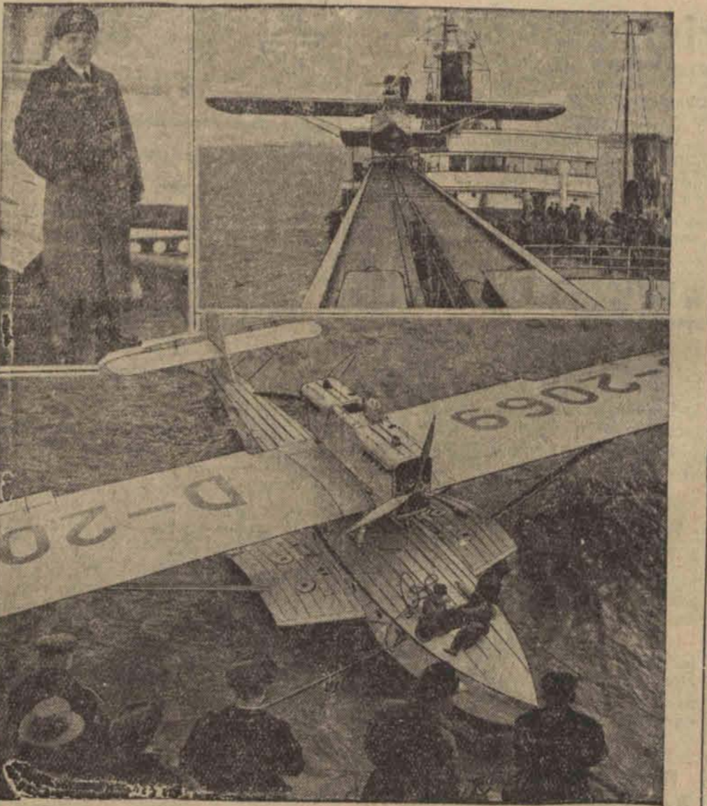
Próby hydroplanu na sztucznej wyspie lotniska Westfalen między Afryką a Ameryką Południową. U góry: 1) Dowódca okrętu lotniska 2) Szyny rozpędowe dla odlotu hydroplanu. U dołu: Hydroplan na wodzie u boku okrętu.
