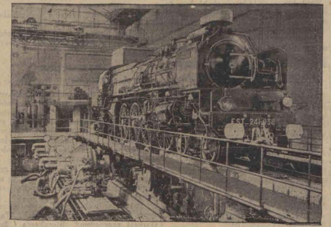
Nowoczesne urządzenie dla próby parowozów w laboratorium fabrycznym.
