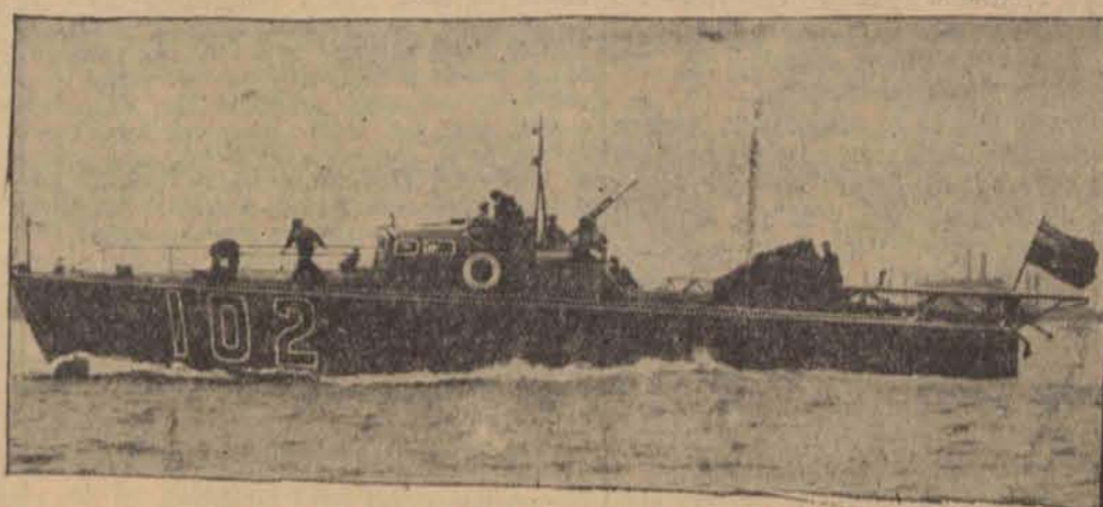
Tysiącny motor pozwala osiągnąć angielskiemu ścigaczowi szybkość 80 km na godzinę. Na pokładzie ścigacza znajdują się wyrzutnia torped i 21 torped, będących groźnym niebezpieczeństwem dla największych pancerników. Mała i szybka łódź jest nieuchwytnym celem dla powolnych okrętów wojennych.
