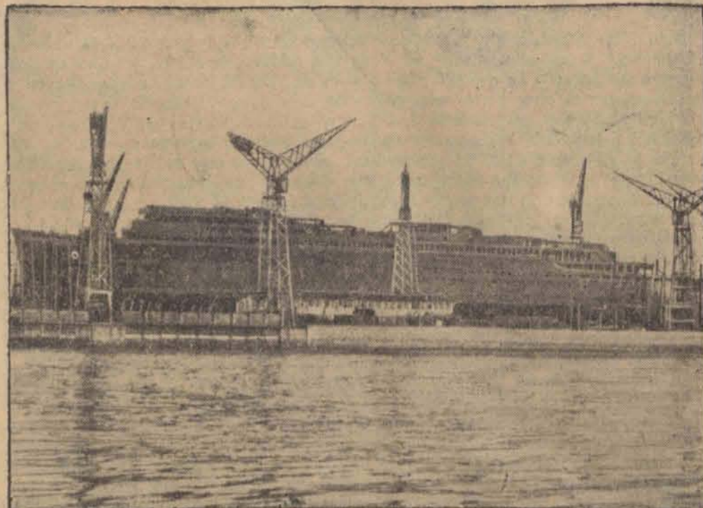
W stoczni St. Nazaire dobiega końca budowa statku pasażerskiego „Pasteur” dla linii południowo-amerykańskiej. Statek ten zastąpi spalony przed kilku laty „Atlantique”. „Pasteur” ma 200 m długości i pojemności 28.500 ton.
