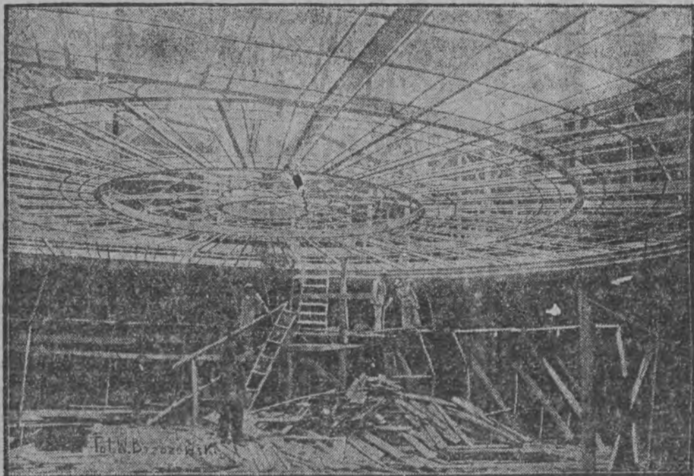
Konstrukcja żelazna szklanego dachu nad nową salą obrad.
