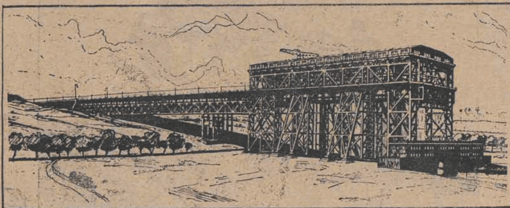
Projekt wielkiego dźwigu okrętowego, który ma być wybudowany w Gdyni ze składek i ofiar, zbieranych przez wojewódzkie oddziały Ligi Morskiej i Riecznej.
