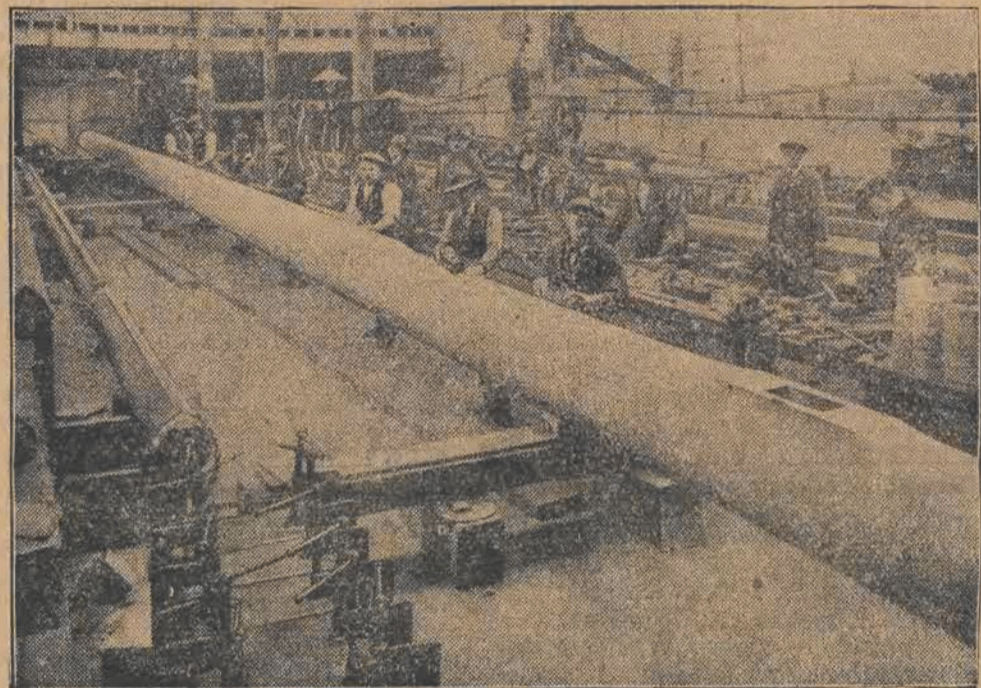
Słynny angielski „król herbaty”, Tomasz Lipton, kazał zbudować sobie olbrzymi jacht, przy którego pomocy pragnie zdobyć t. zw. „puhar Ameryki”, nagrodę za najszybsze przebycie oceanu. — Na zdjęciu: obrabianie głównego masztu dla tego jachtu, który zwać się będzie „Shamrock V”.
