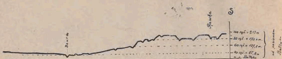
Przekrój wzdłuż południka 10°21' od Pulkowa 8 klm. na wschód od Łowicza. Stosunek skał pionowej do skał poziomej 1:40.
